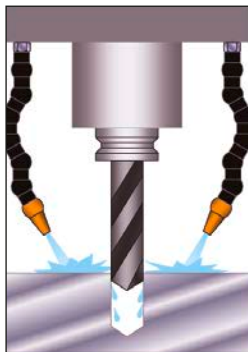
Chłodzenie natryskowe
