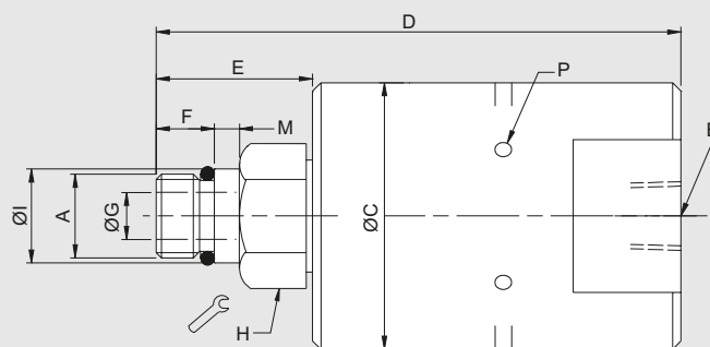
Przylącze osiowe (seria 7000)
