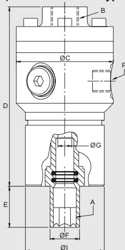
Przyłącze osiowe (1109-710-717 na zdjęciu)
