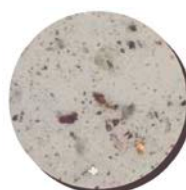
Niedozwolone (ISO 21/19/17 w powiększeniu 100x)
